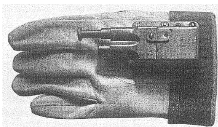
Slika 3.11: Naprava na en strel, pritrjena na usnjeno rokavico, ki strelja med prsti
